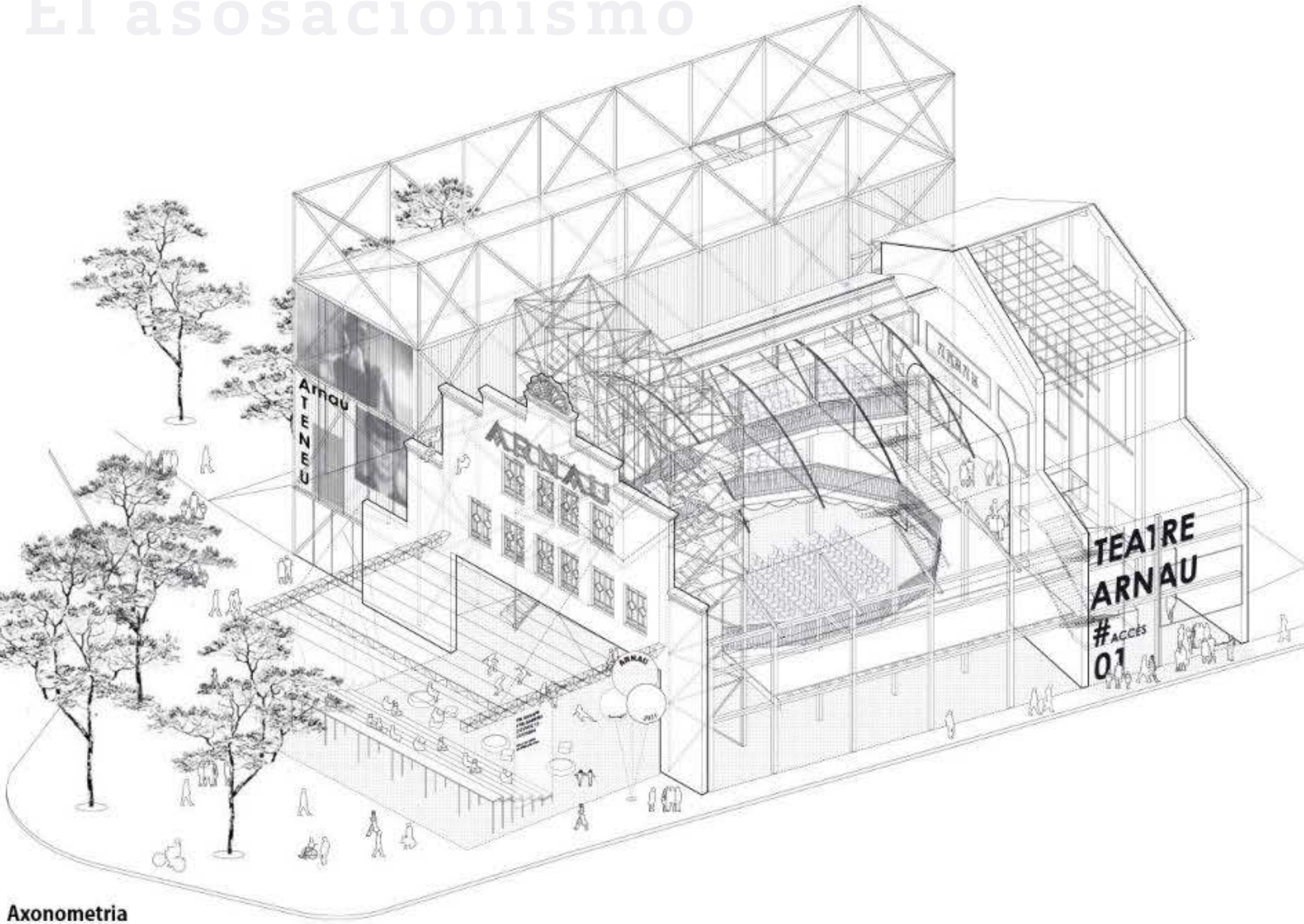
Axonometria Teatre Arnau
